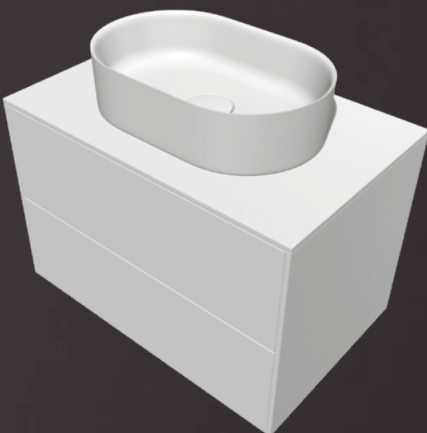
80 | WBT80001 800x515x540 мм
